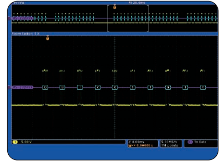
▶ RS-232 버스를 통과하는 특징 데이터 패킷 트리거링
